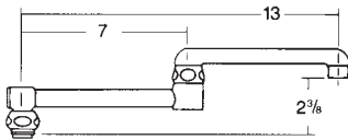
17441 E3 aerator, E2 outlet available
