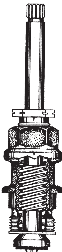
PRICE PFISTER PP319 Diverter stem
